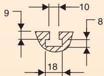
T-10 'T' SLOT
